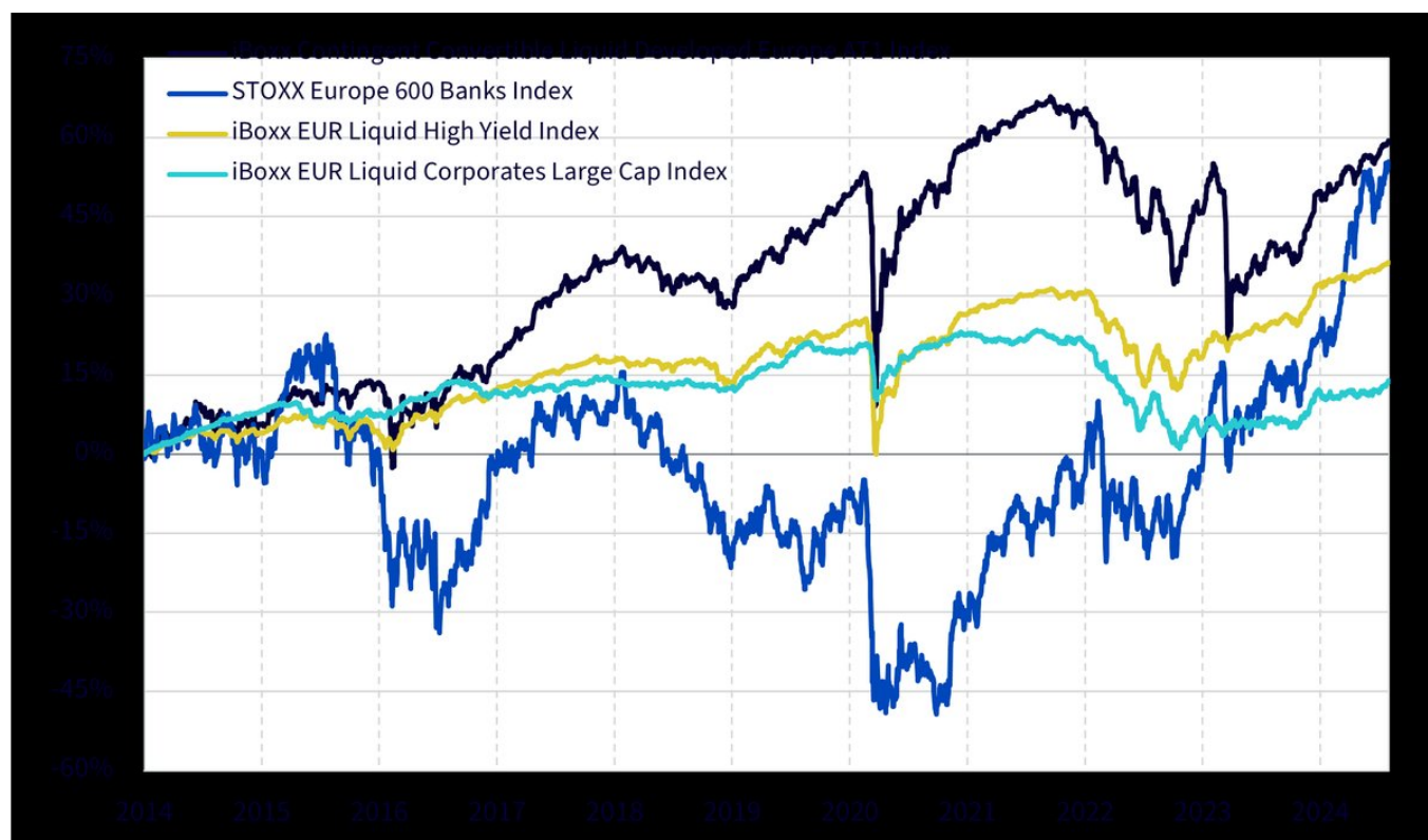
Figura 2: Rendimenti cumulati
